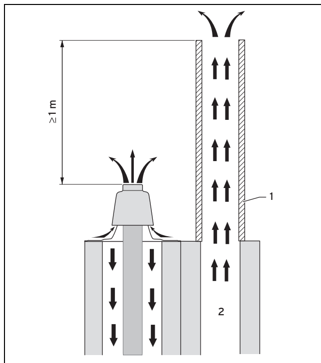
1 Насадка димаря
